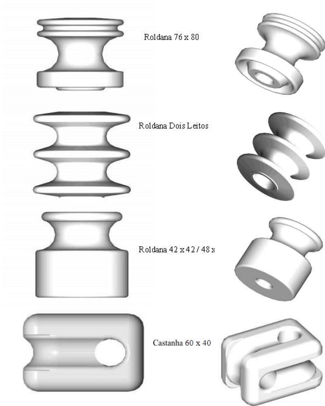
FIGURA 65 - ISOLADORES
