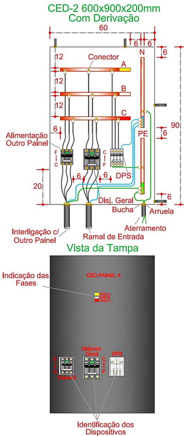
FIGURA 48 - LAY-OUT DE CED-2 (600X900X200 MM) COM DERIVAÇÃO
