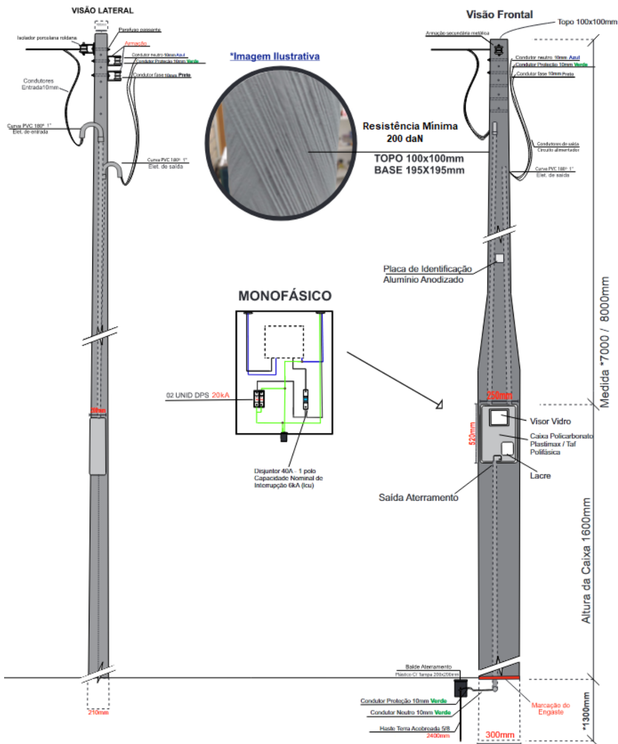
FIGURA 59 - POSTE FIBRA DE VIDRO COM CAIXA DE MEDIÇÃO MONOFÁSICA INCORPORADA
