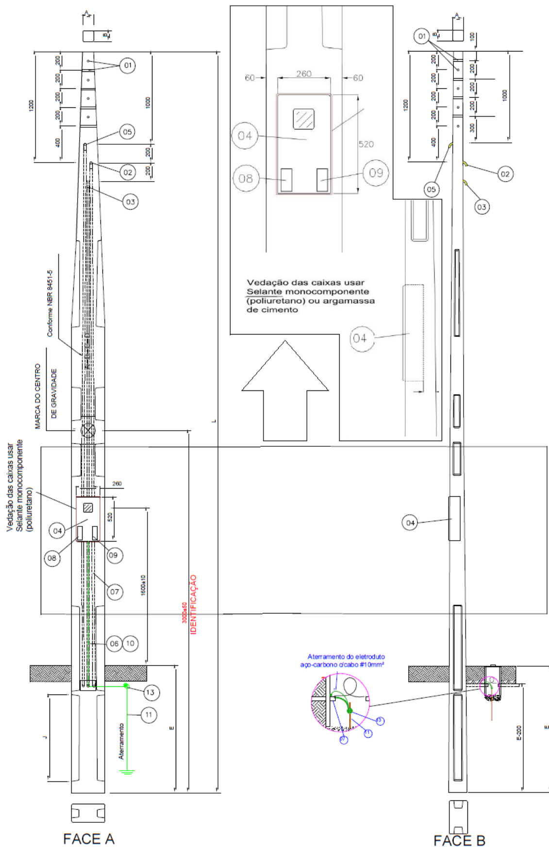
FIGURA 58 - POSTE COM UMA CAIXA DE MEDIÇÃO POLIFÁSICA INCORPORADA
