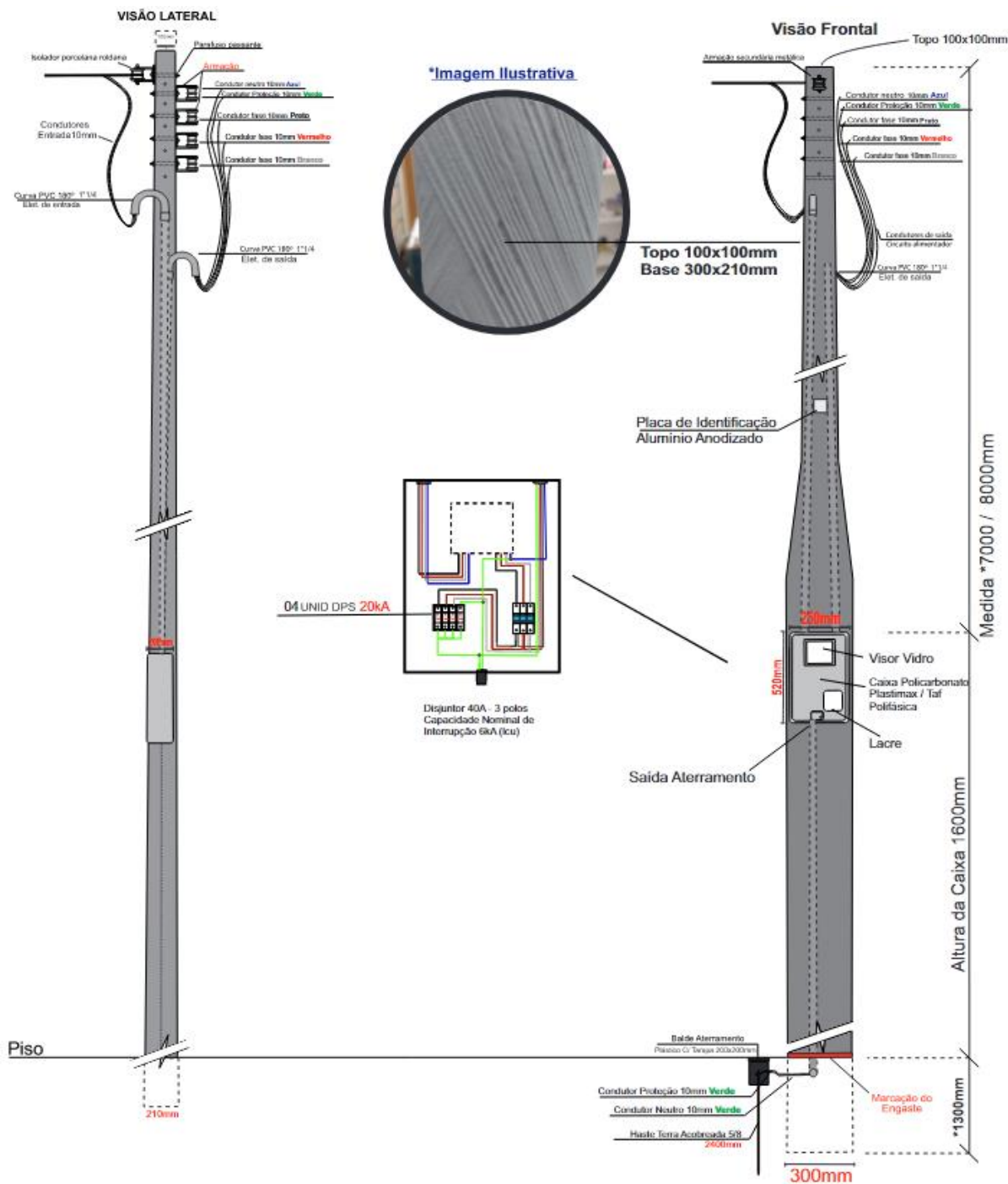
FIGURA 60 - POSTE FIBRA DE VIDRO COM CAIXA DE MEDIÇÃO POLIFÁSICA INCORPORADA
