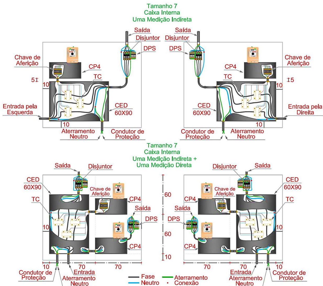
FIGURA 39 - MONTAGEM CAIXAS PARA MEDIDORES POLIFÁSICOS MEDICÇÃO INDIRETA
