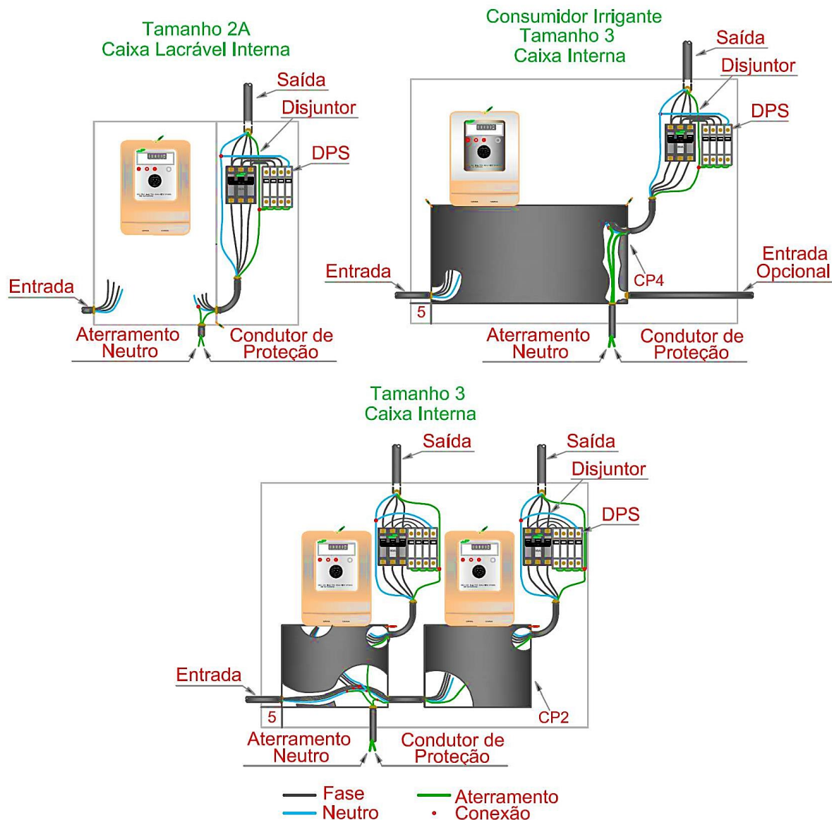
FIGURA 38 - MONTAGEM CAIXAS PARA MEDIDORES POLIFÁSICOS COM MEDIÇÃO DIRETA
