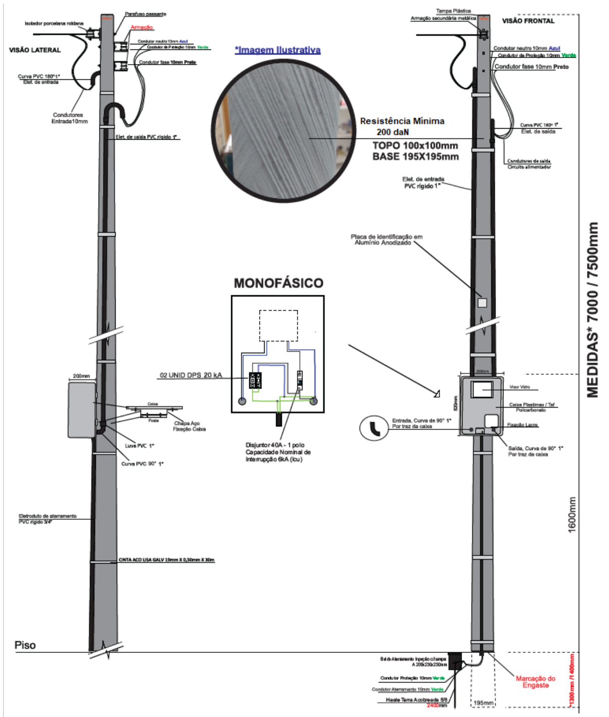
FIGURA 61 - POSTE FIBRA DE VIDRO COM CAIXA DE SOBREPOR MONOFÁSICA
