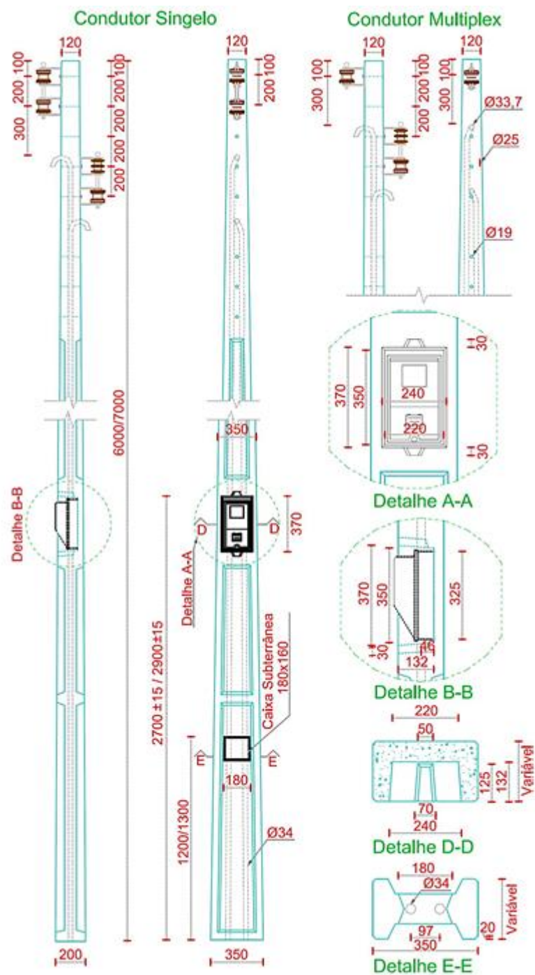
FIGURA 57 - POSTE PARTICULAR DE CONCRETO ARMADO COM CAIXA DE MEDIÇÃO MONOFÁSICA ACOPLADA
