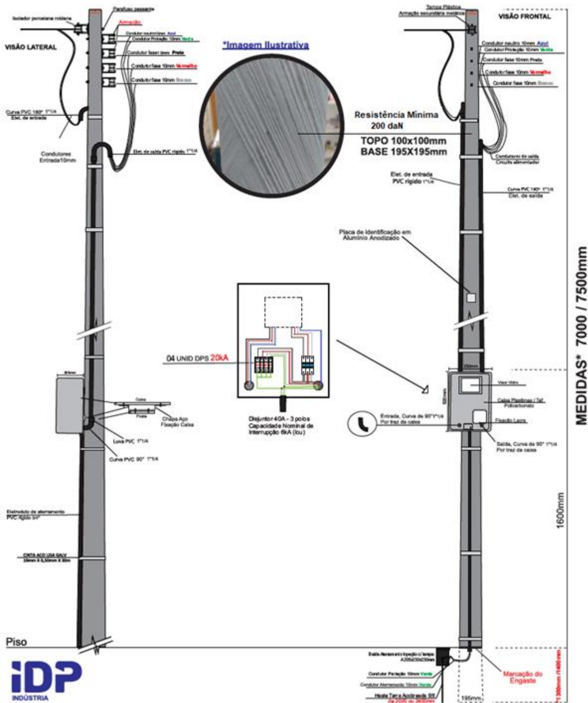
FIGURA 62 - POSTE FIBRA DE VIDRO COM CAIXA DE SOBREPOR POLIFÁSICA
