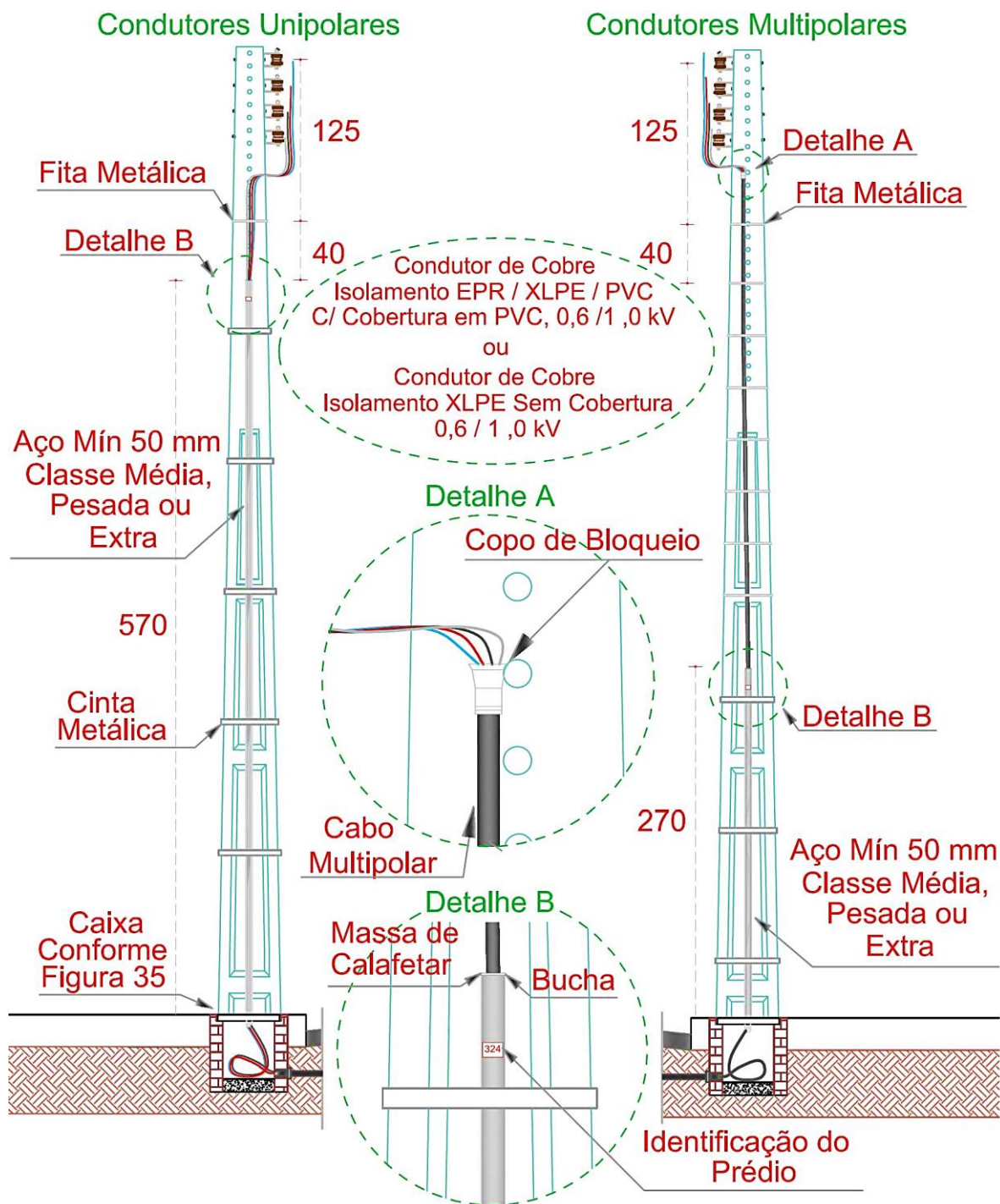
FIGURA 30 - FIXAÇÃO DOS CONDUTORES DE ENTRADA SUBTERRÂNEA NO POSTE
