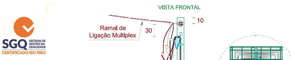
FIGURA 15 - ENTRADA DE ENERGIA COM MEDIÇÃO INSTALADA EM MURO OU MURETA FRONTAL COM GRADE E CADEADO PADRÃO
