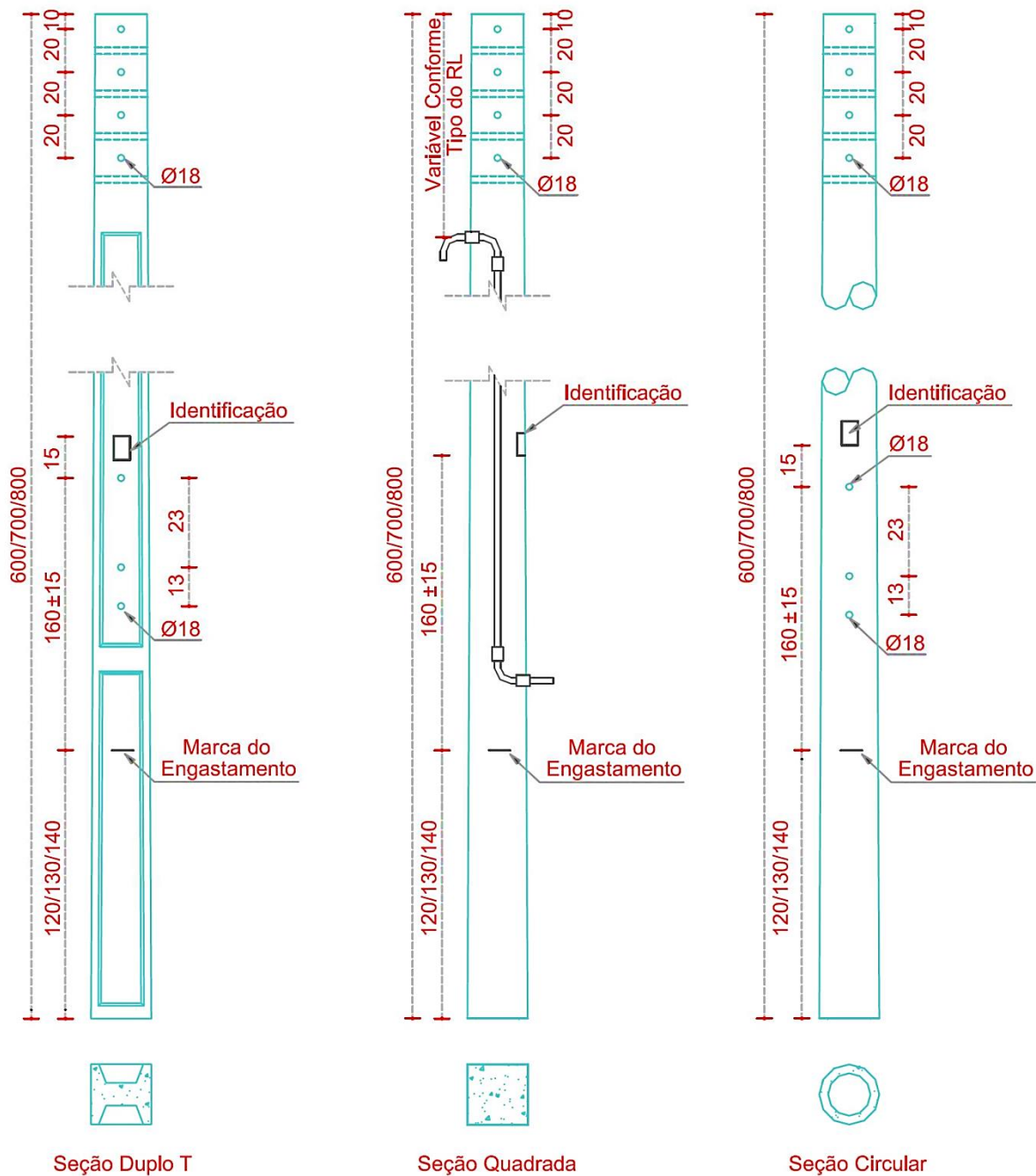
FIGURA 55 - POSTE PARTICULAR DE CONCRETO ARMADO
