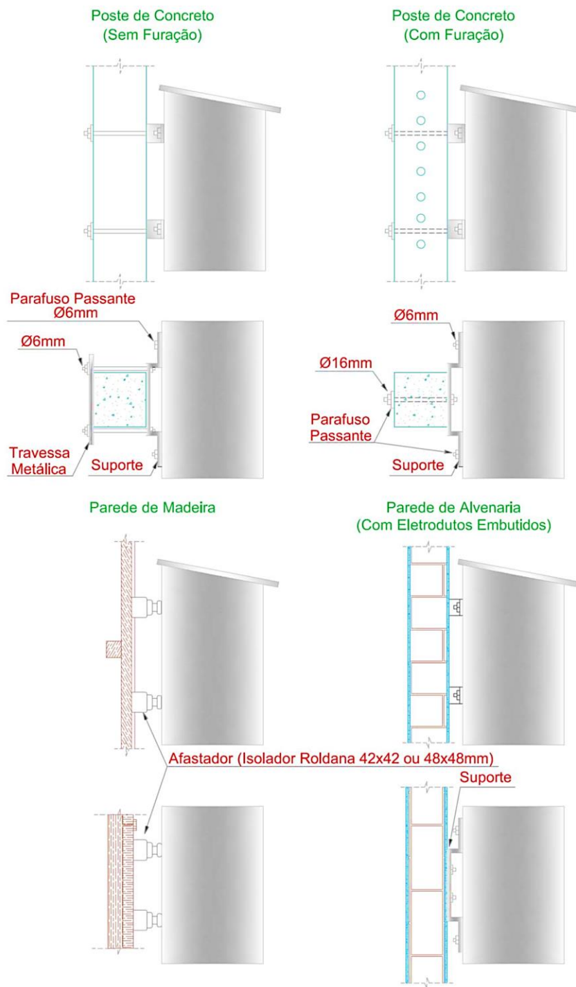
FIGURA 34 - FIXAÇÃO DE CAIXAS PARA MEDIDORES EM MADEIRA E ALVENARIA
