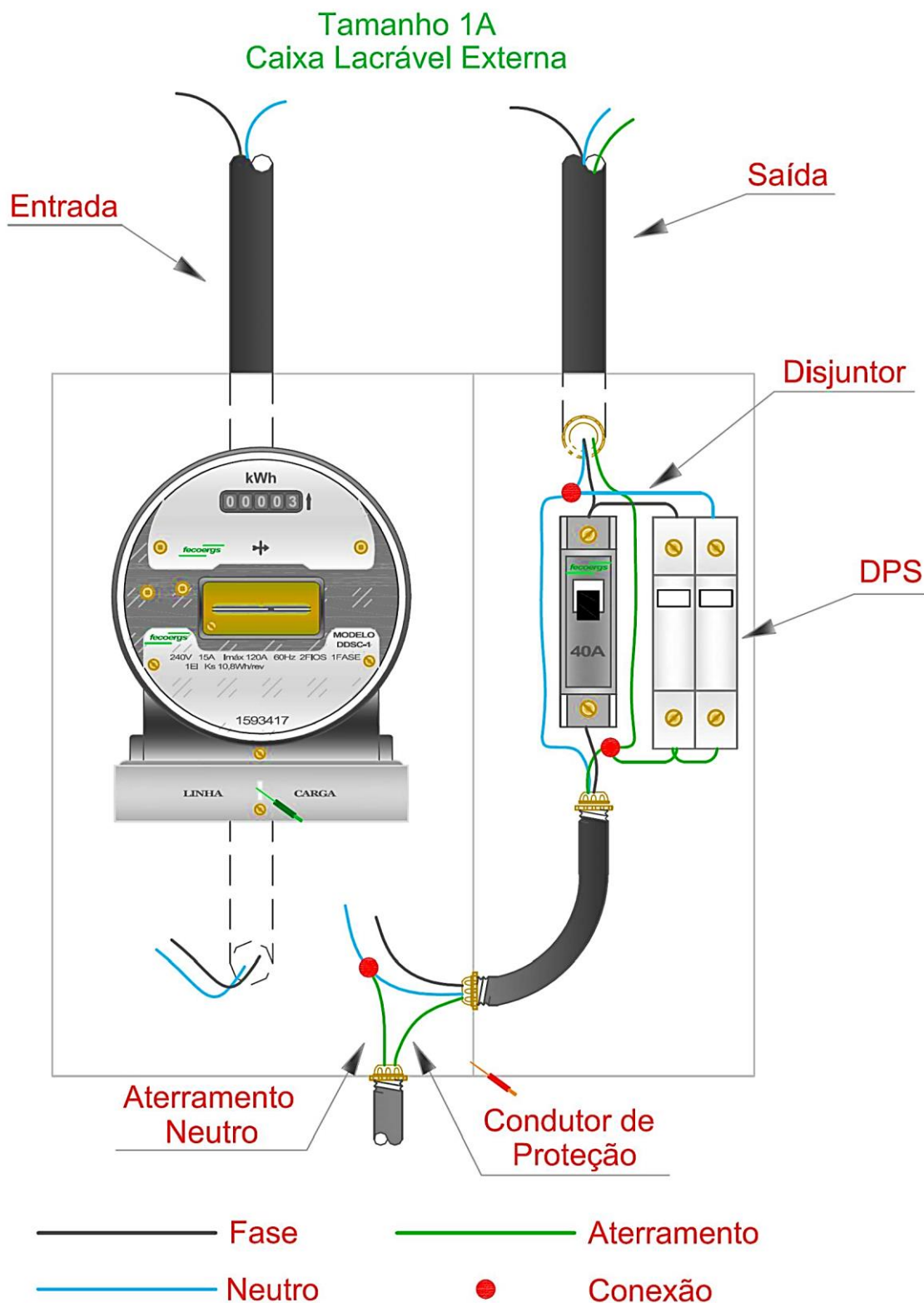
FIGURA 38 - MONTAGEM DAS CAIXAS PARA MEDIDORES MONOFÁSICOS
