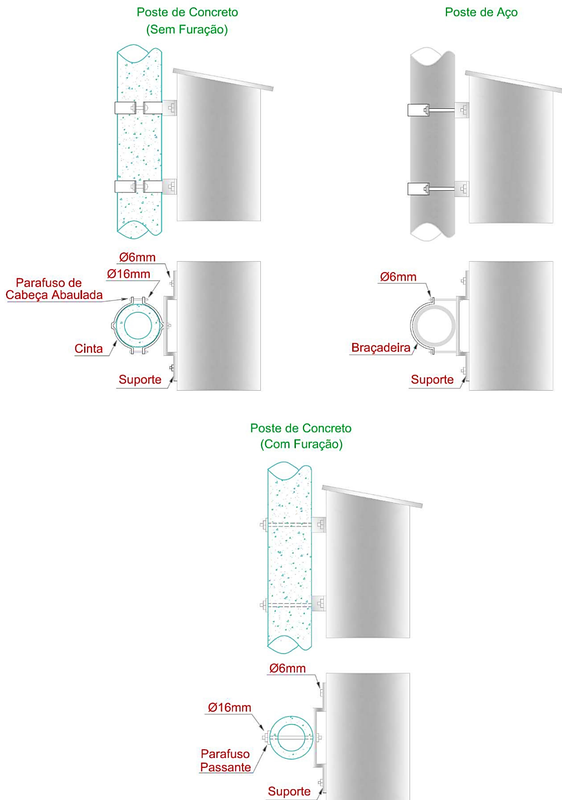
FIGURA 33 - FIXAÇÃO DE CAIXAS PARA MEDIDORES EM POSTES
