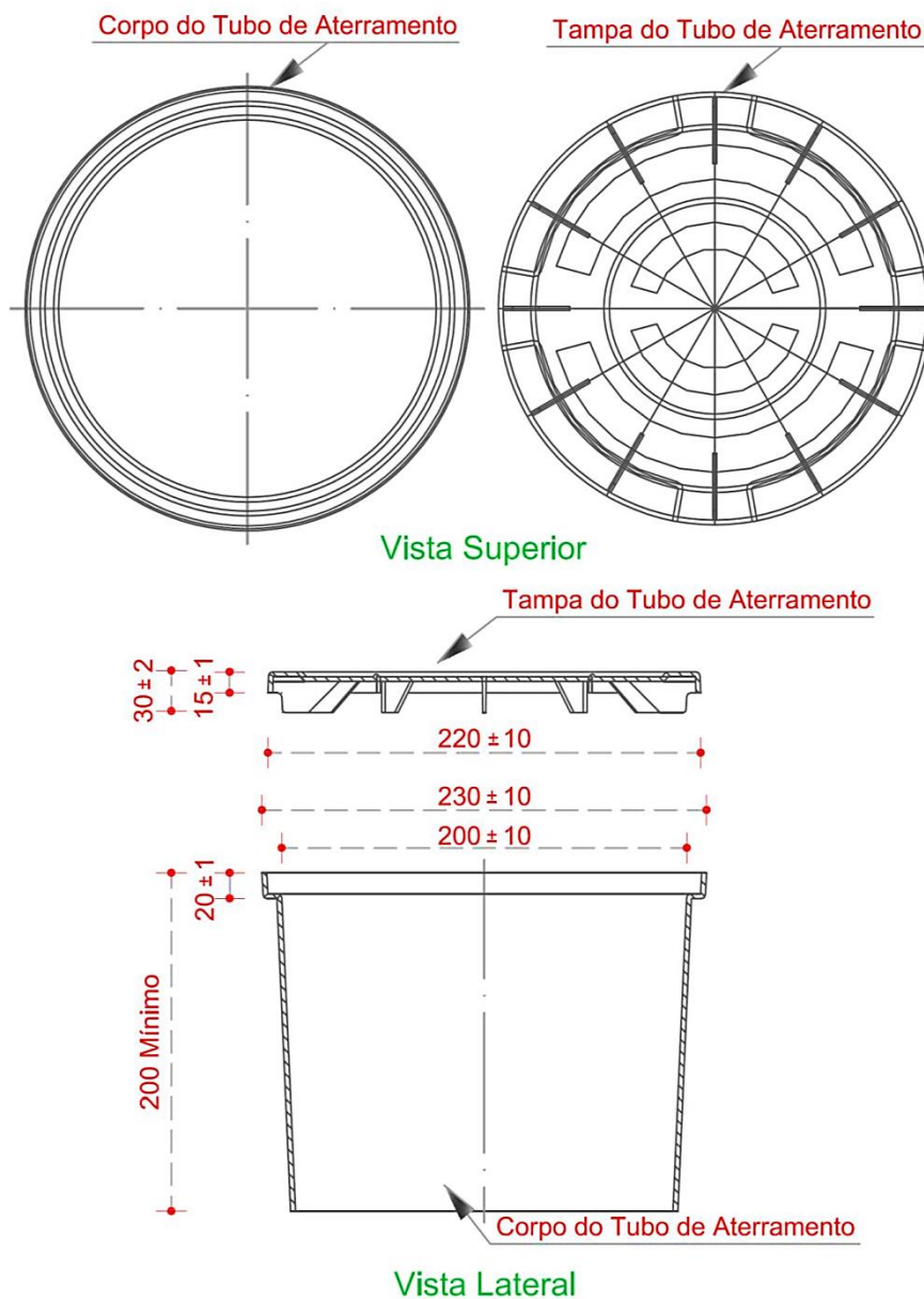
FIGURA 65 – TUBO PARA ATERRAMENTO
