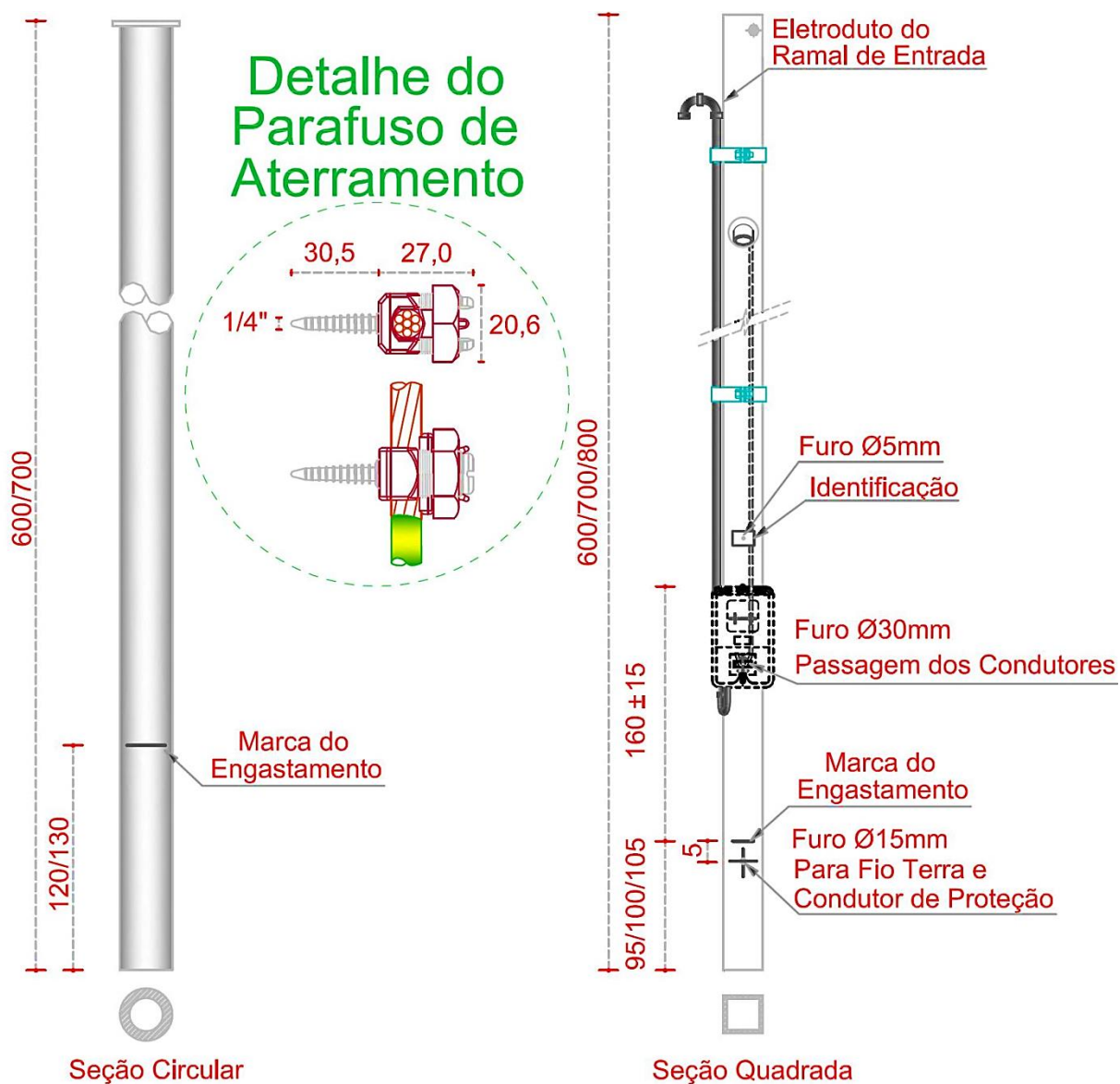
FIGURA 56 - POSTE PARTICULAR DE AÇO SEM E COM CAIXA DE MEDIÇÃO ACOPLADA
