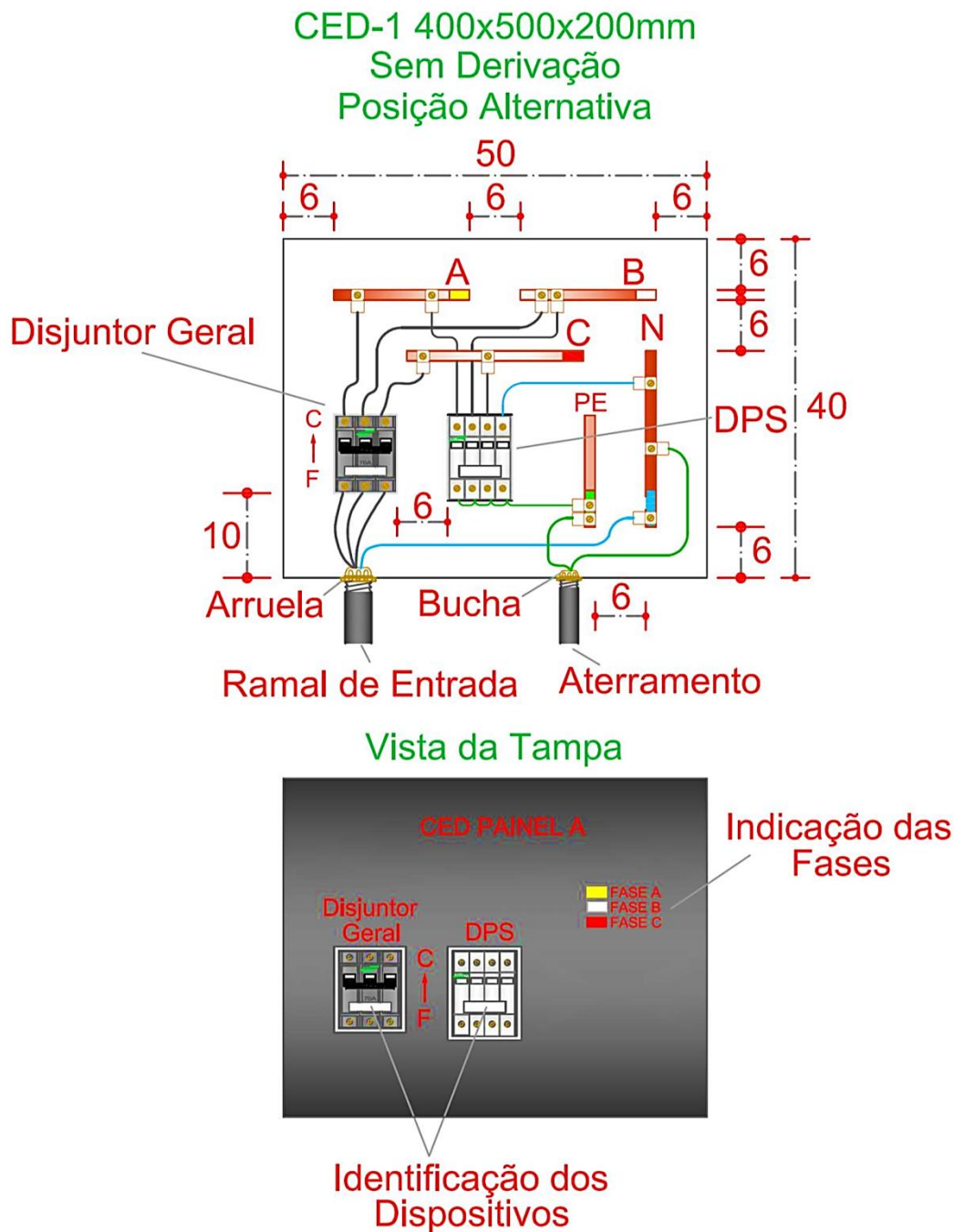
FIGURA 47 - LAY-OUT DE CED-1 (400X500X200 MM) SEM DERIVAÇÃO EM POSIÇÃO ALTERNATIVA
