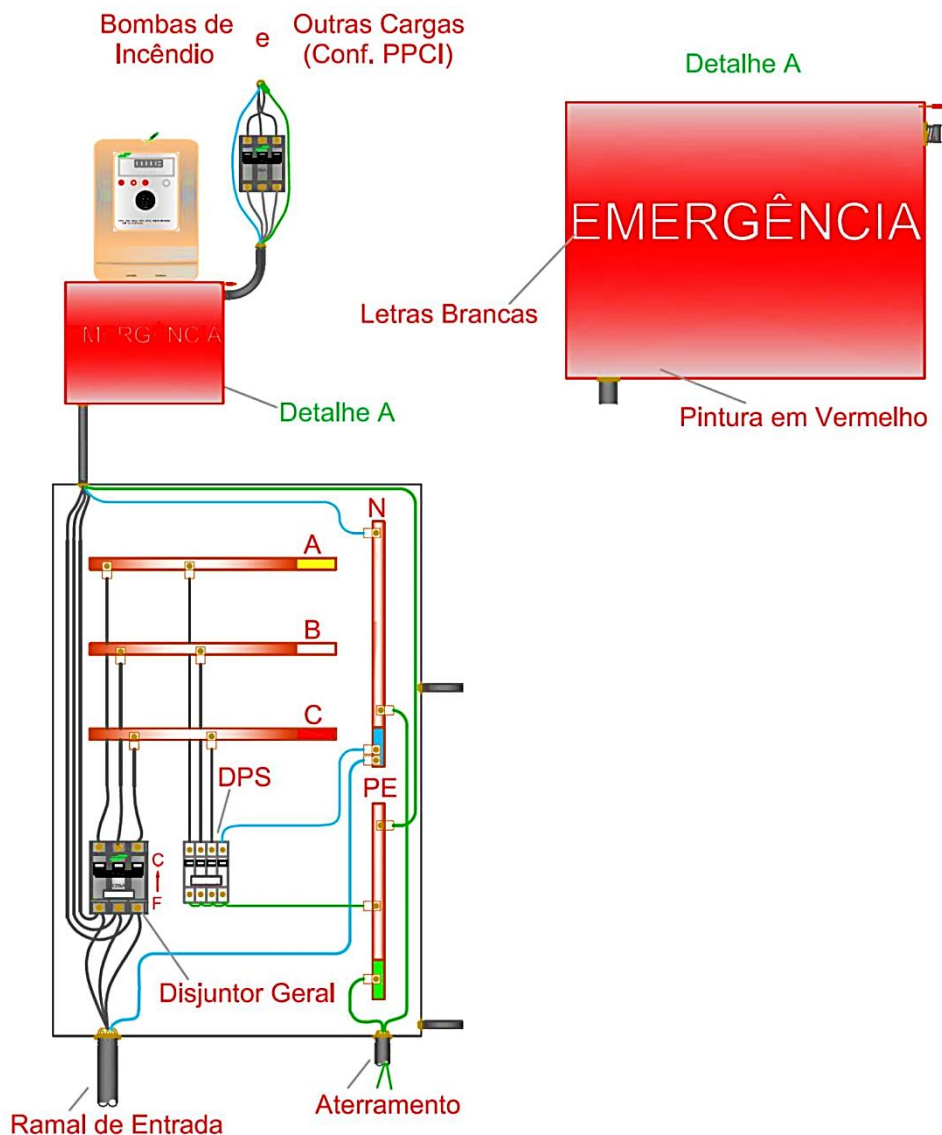
FIGURA 54 - SISTEMA DE EMERGÊNCIA
