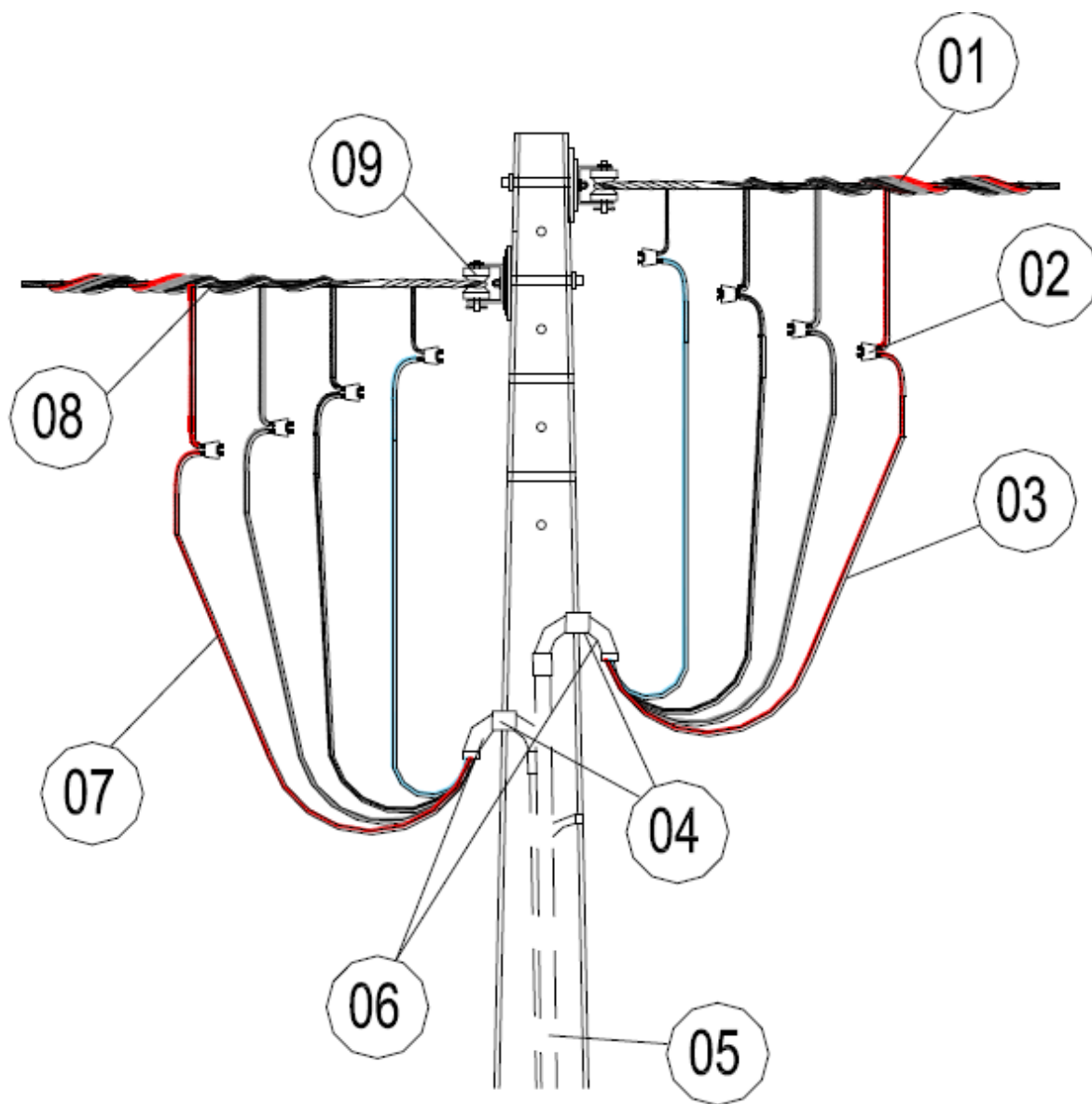
FIGURA 61 – DETALHE ANCORAGEM DO RAMAL DE LIGAÇÃO E CONEXÕES
