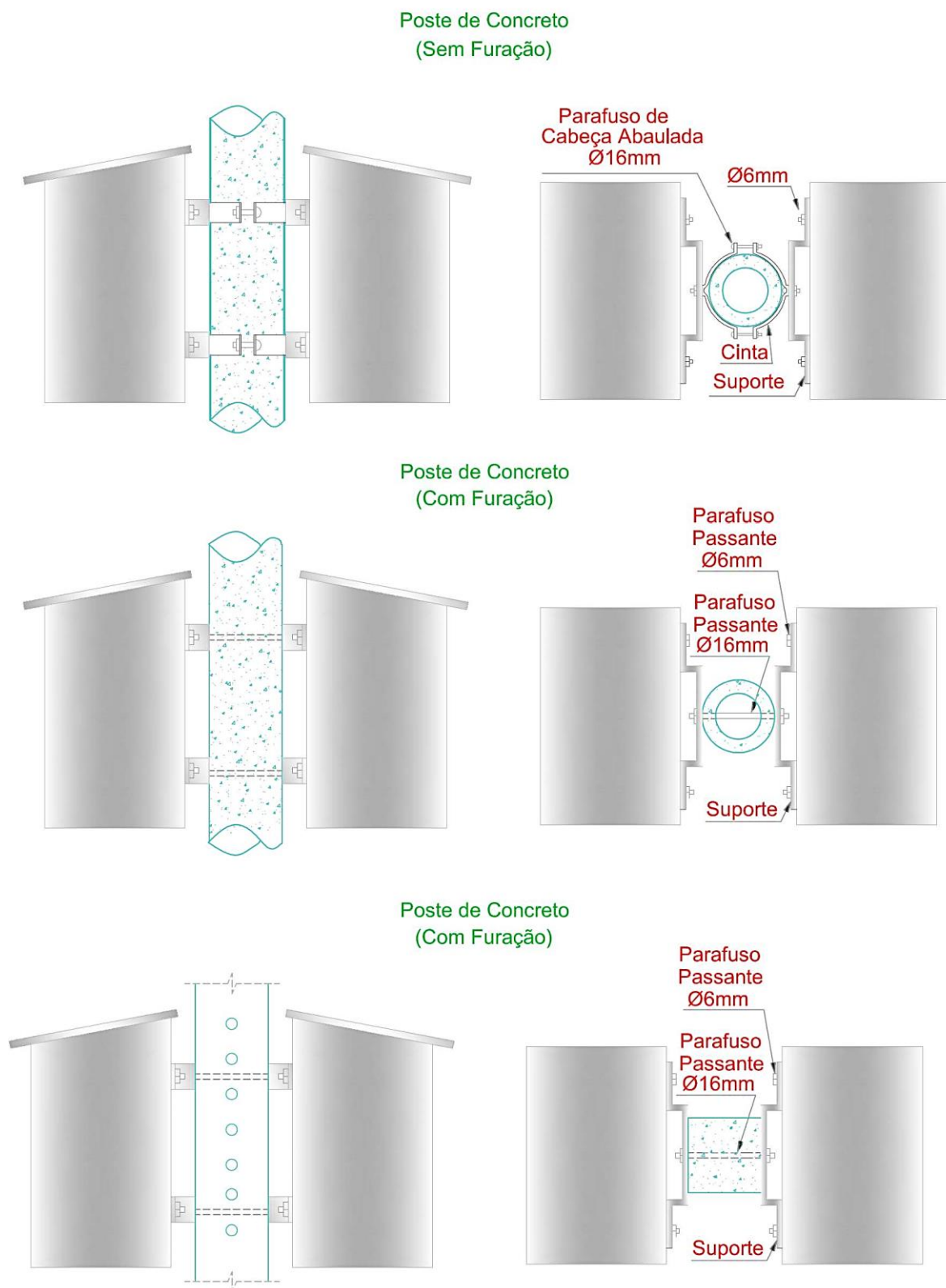
FIGURA 36 - FIXAÇÃO DE CAIXAS PARA MEDIDORES - DUAS CAIXAS NO MESMO POSTE
