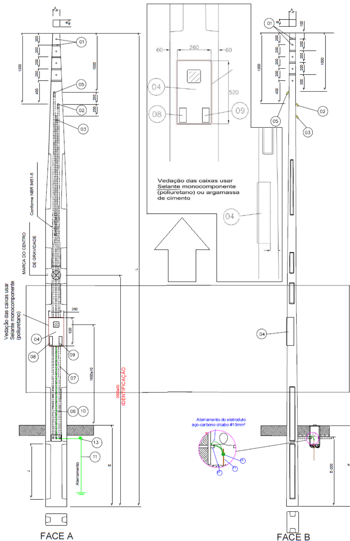
FIGURA 60 - POSTE COM UMA CAIXA DE MEDIÇÃO POLIFÁSICA INCORPORADA
