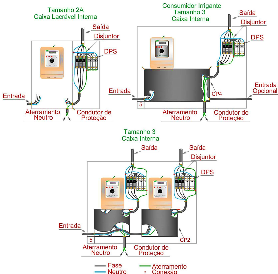
FIGURA 39 – MONTAGEM CAIXAS PARA MEDIDORES POLIFÁSICOS COM MEDIÇÃO DIRETA
