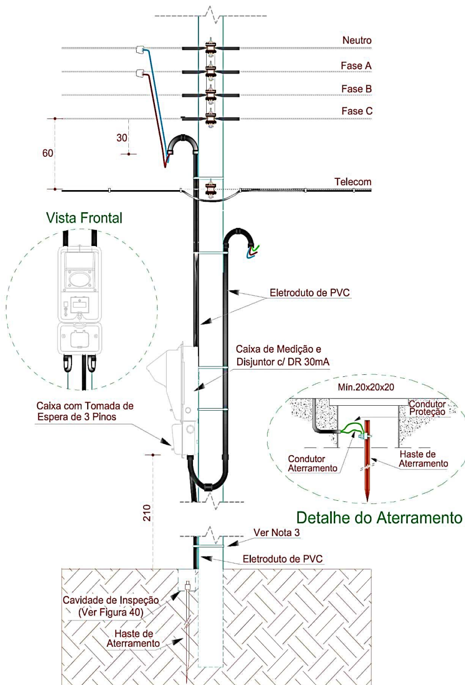
FIGURA 24 - MEDIÇÃO FIXADA NO POSTE DA CONCESSIONÁRIA – CASOS ESPECIAIS – CAIXA COM TOMADA DE ESPERA DE 3 PINOS
