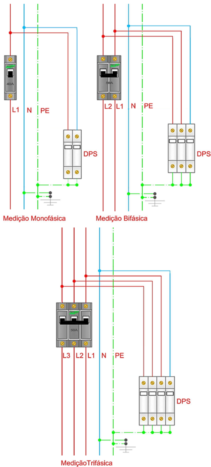
FIGURA 50 - CONEXÃO DE DPS
