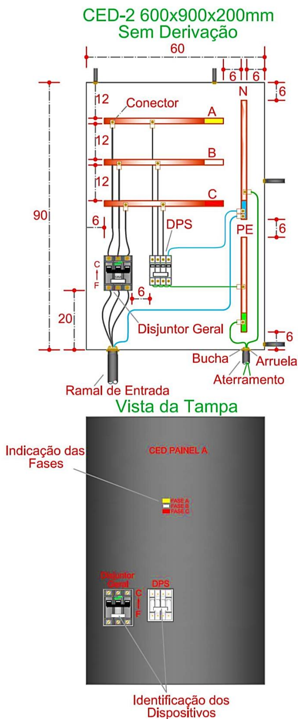
FIGURA 48 - LAY-OUT DE CED-2 (600X900X200 MM) SEM DERIVAÇÃO
