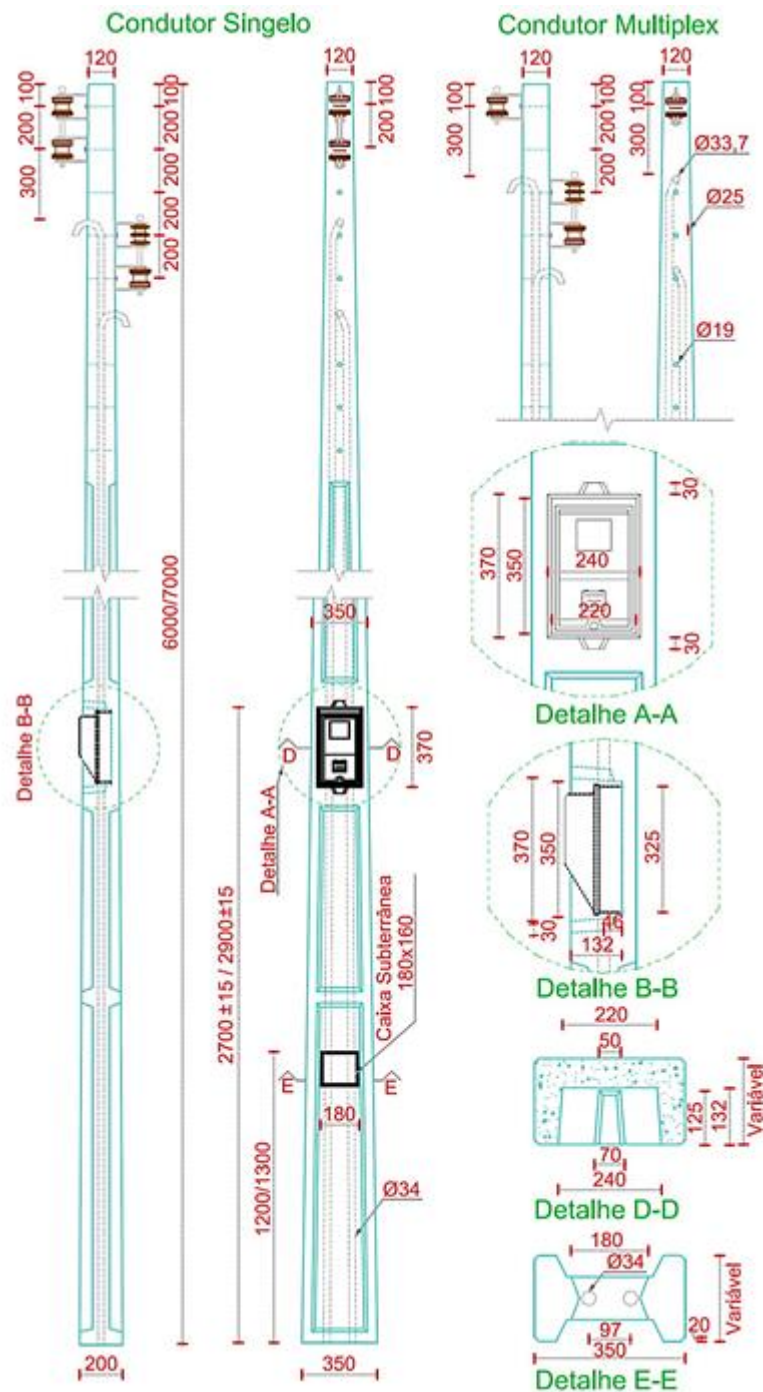
FIGURA 59 - POSTE PARTICULAR DE CONCRETO ARMADO COM CAIXA DE MEDIÇÃO MONOFÁSICA ACOPLADA
