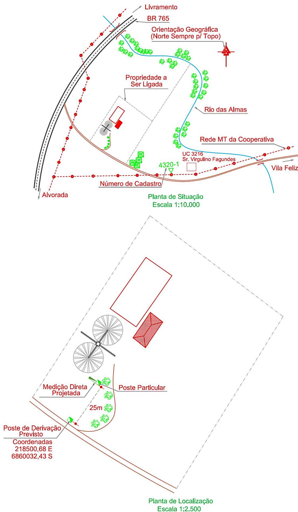
FIGURA 52 - PLANTA DE SITUAÇÃO E PLANTA DE LOCALIZAÇÃO EM ÁREA RURAL
