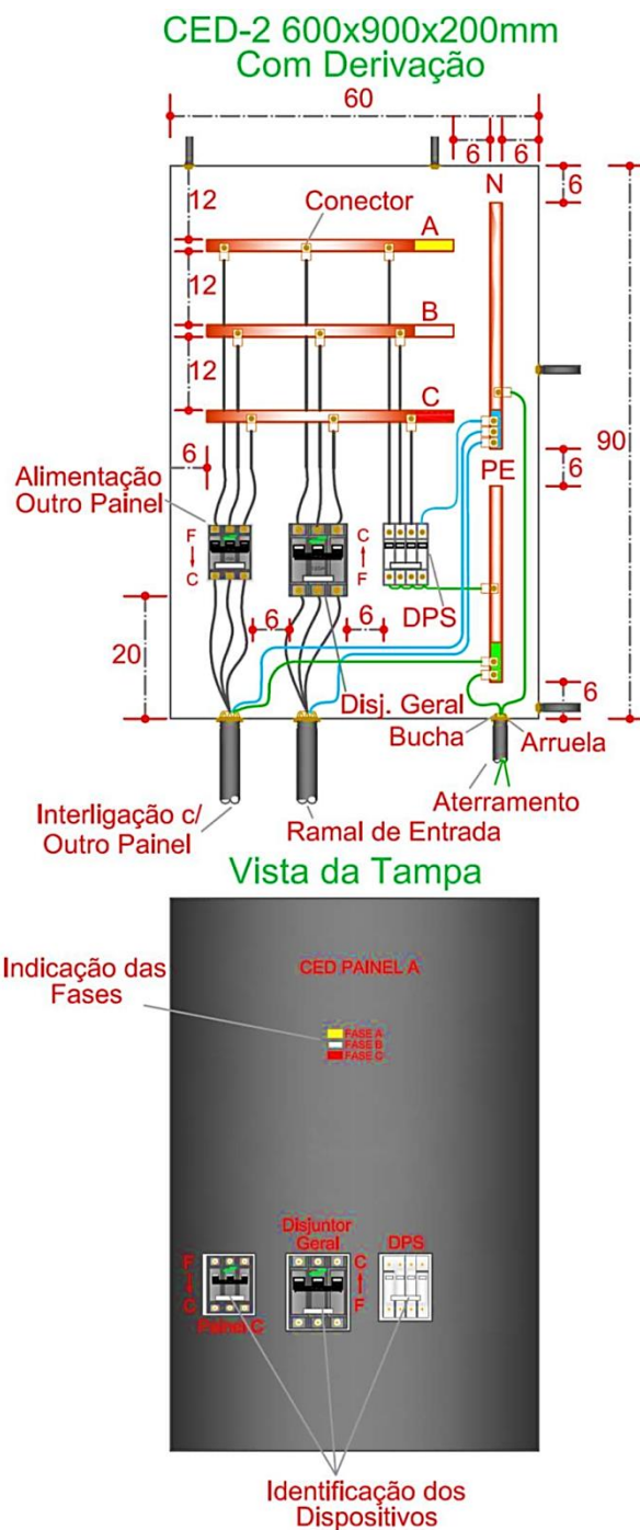
FIGURA 49 - LAY-OUT DE CED-2 (600X900X200 MM) COM DERIVAÇÃO
